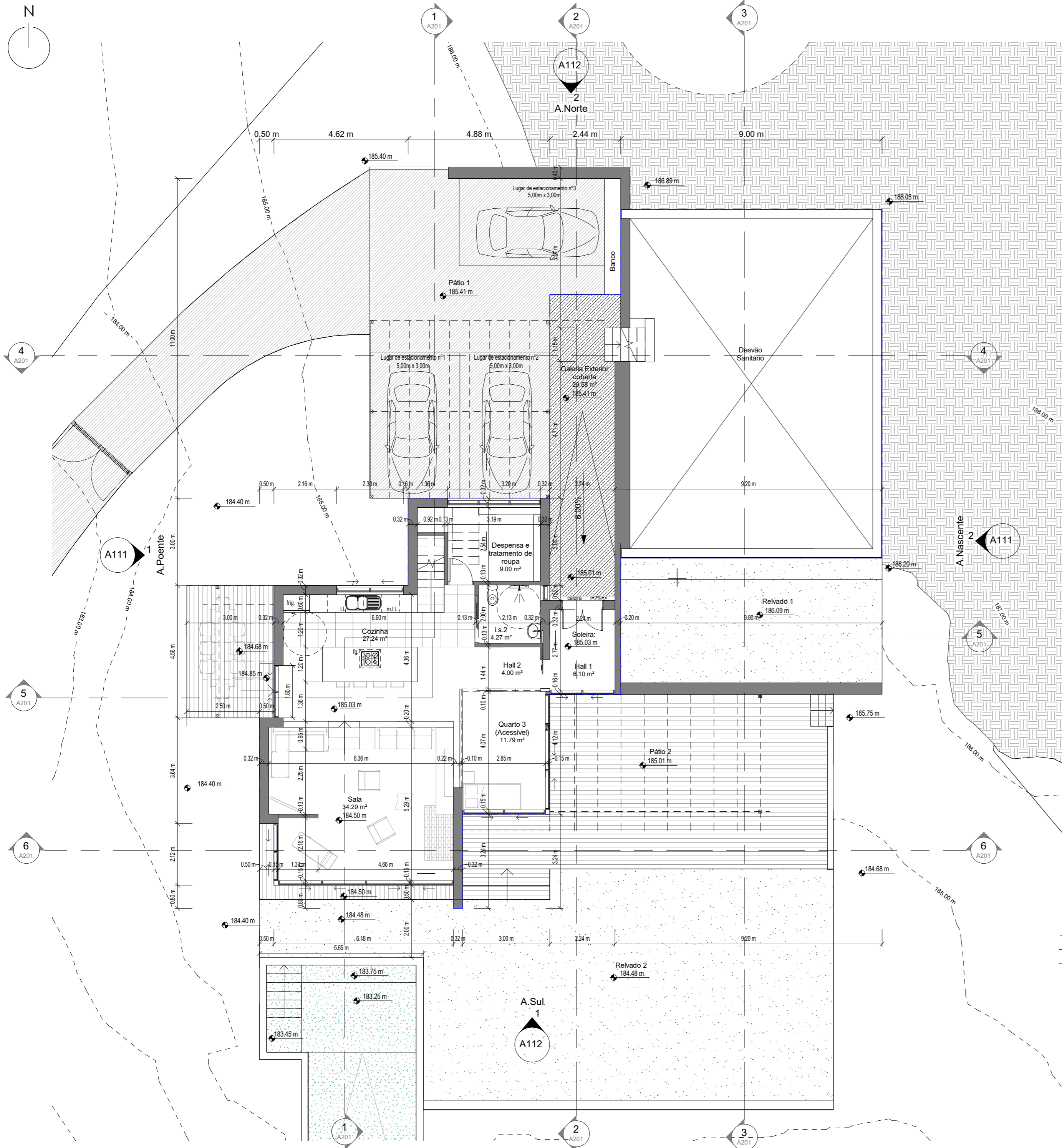
1 Piso 1 1 : 100
